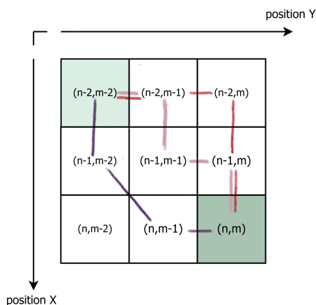
FIGURE 7.6 – Chevauchement des sous-problèmes - plusieurs chemins éventuels
