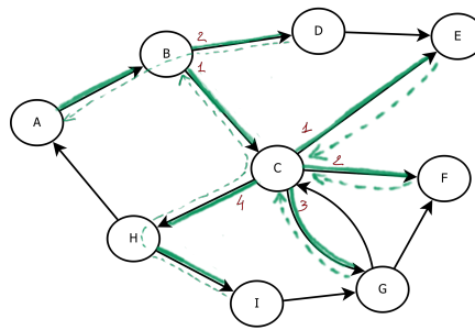
Parcours et distances
