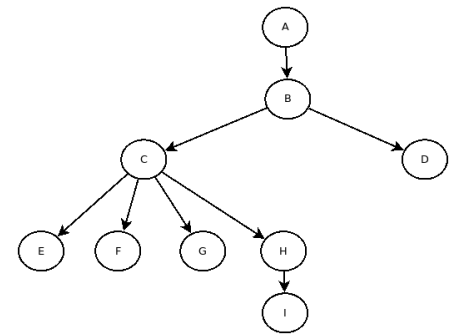
Graphe du parcours
