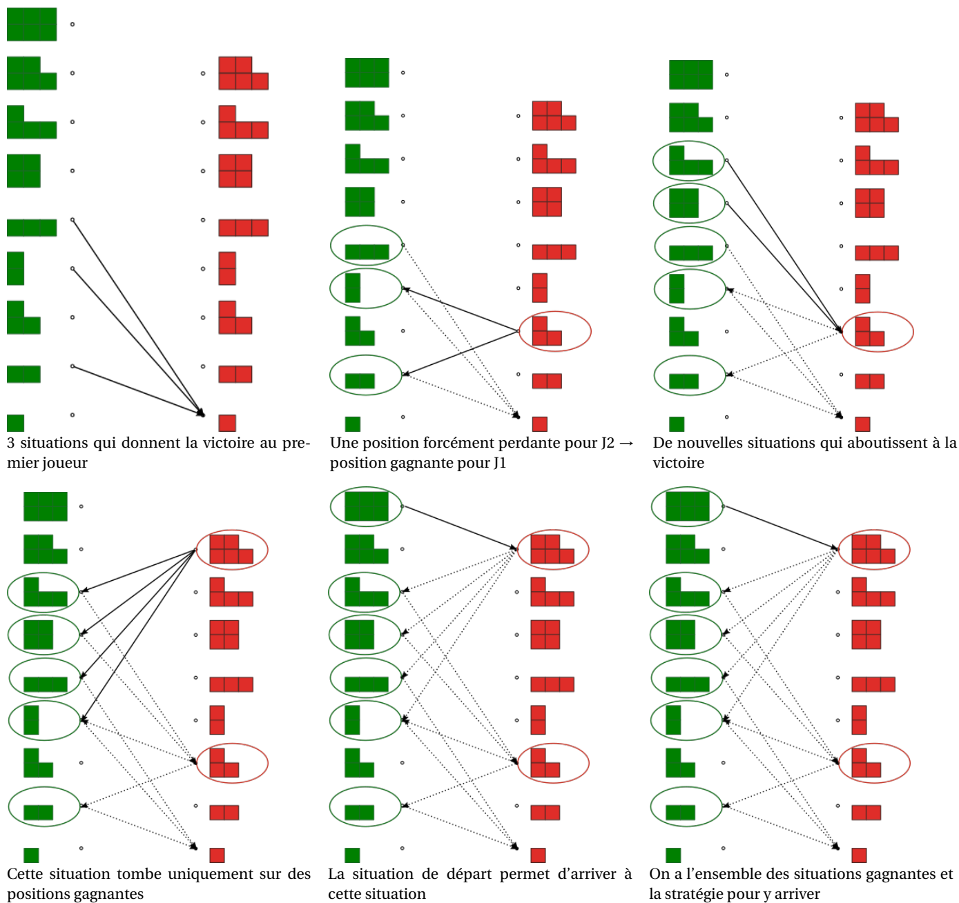
Illustration du calcul des positions gagnantes dans le jeu de chomp
